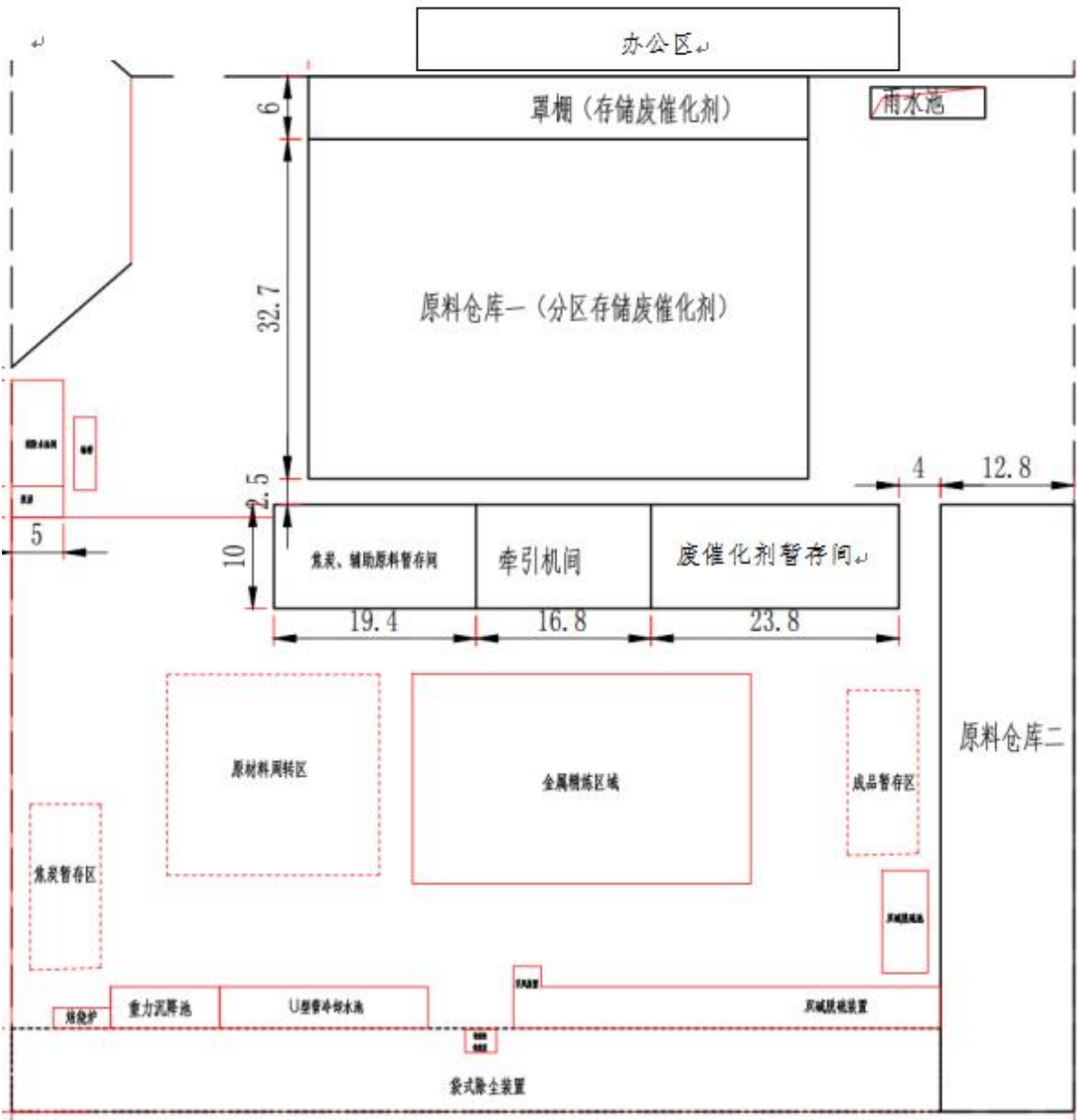
图 3.2-1 厂区平面布置图
