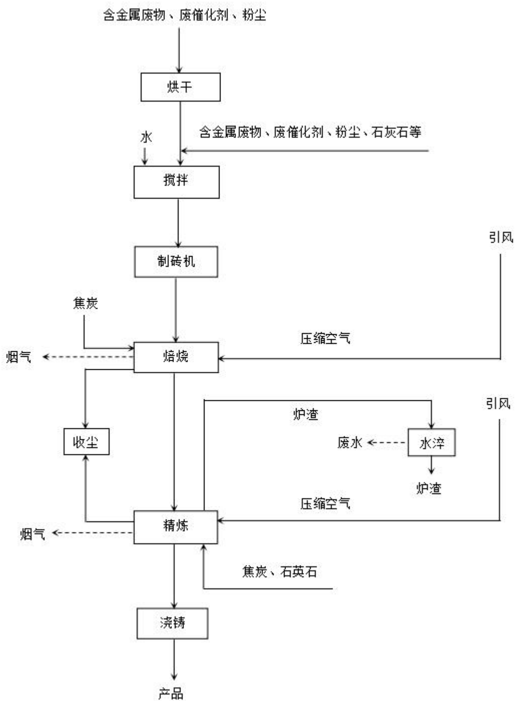
图 2.4-1 氧化锌工艺流程图
